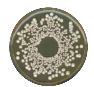
Saccharomyces cerevisiae
